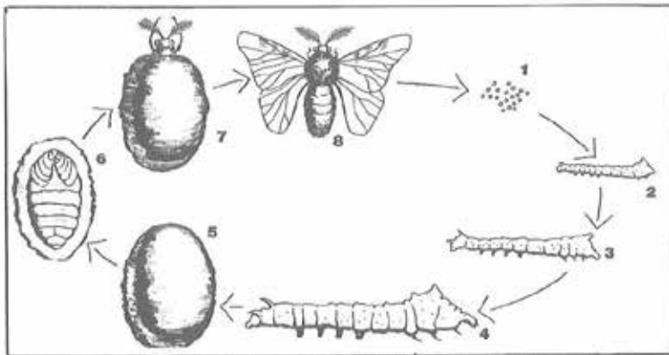
ՇԵՐԱՄԻ ԹԻԹԵՆՆԻԿԻ ԿԵԱՆՔԻ ՇՐՋԱՆԸ: 1- ձուեր 2.3.4- թրթուր 5.6.7- հարսնուկ 8- միջատ
